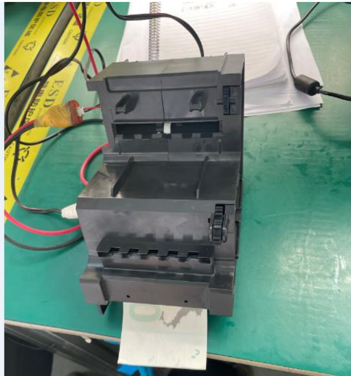
5. 出钱口塞 ITL NOTE 一张, 卡纸, 不出纸, 出纸慢检查齿轮是否漏装。
