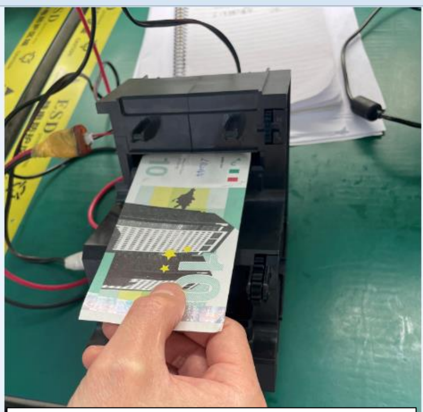
4. 进钱口塞 ITL NOTE 一张,
